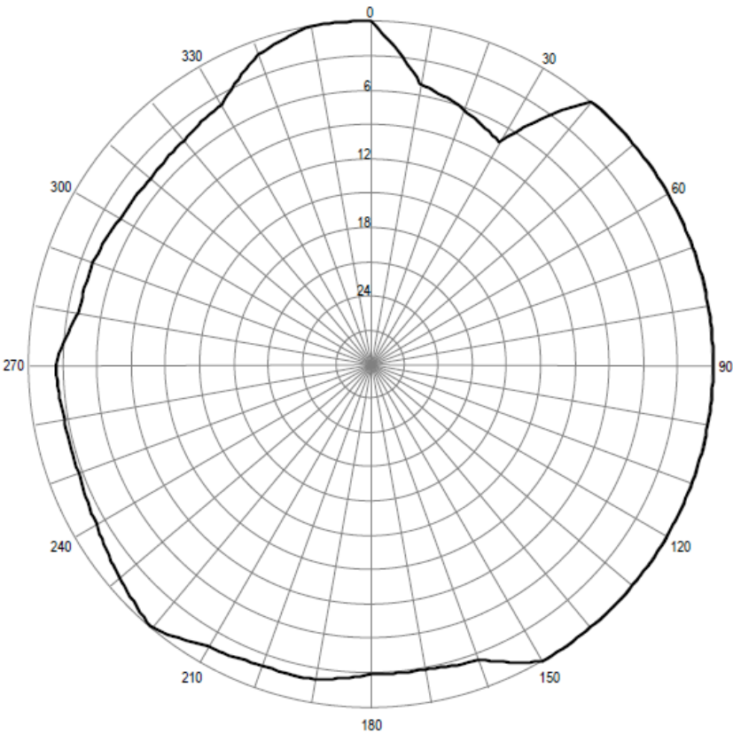
Pozioma charakterystyka promieniowania anteny stacji Warszawa Varso 93,30 MHz
